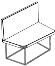
SOFÁ ESQUERDO CABINE 1 E 2 LUGARES 800X450X450MM
