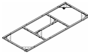
RODAPÉ METÁLICO COM RODÍZIOS CABINE 02 LUGARES
