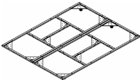
RODAPÉ METÁLICO COM RODÍZIOS CABINE 04 LUGARES
