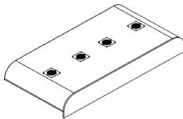
MÓDULO SUPERIOR ORGÂNICO CABINE 02 LUGARES 1850X900X260MM
